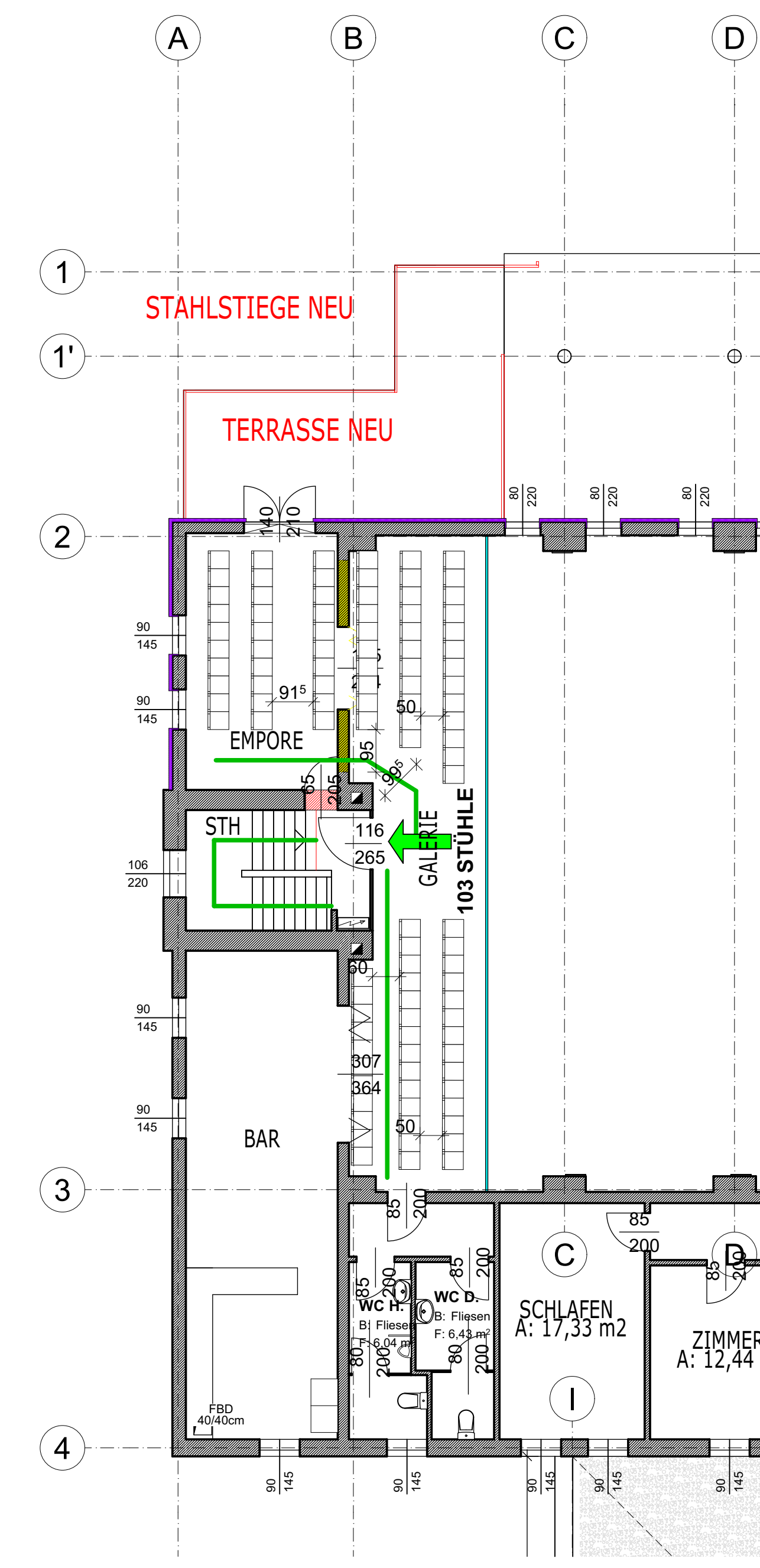
OBERGESCHOSS 1:100
