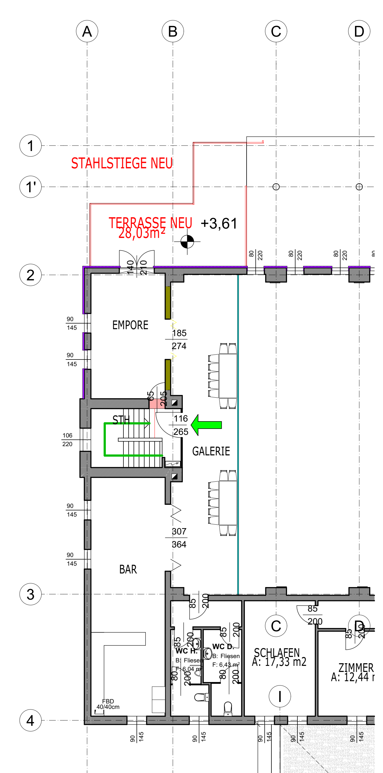
OBERGESCHOSS 1:100
